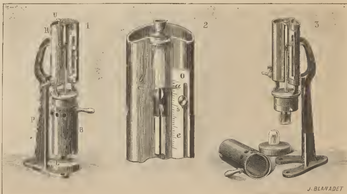
Fig. 4. Determinación de la cantidad de alcohol. - Ebulloscopio de destilador móvil de M. Benevolo. - 1. Vista del aparato en conjunto. - 2. Detalle del cursor en mayor escala. - 3. El aparato desmontado
